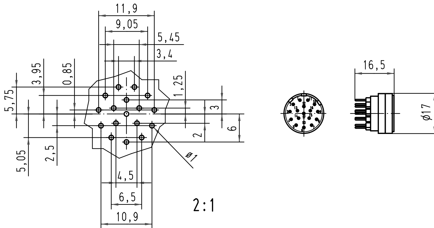
Lochbild/pinhole pattern
