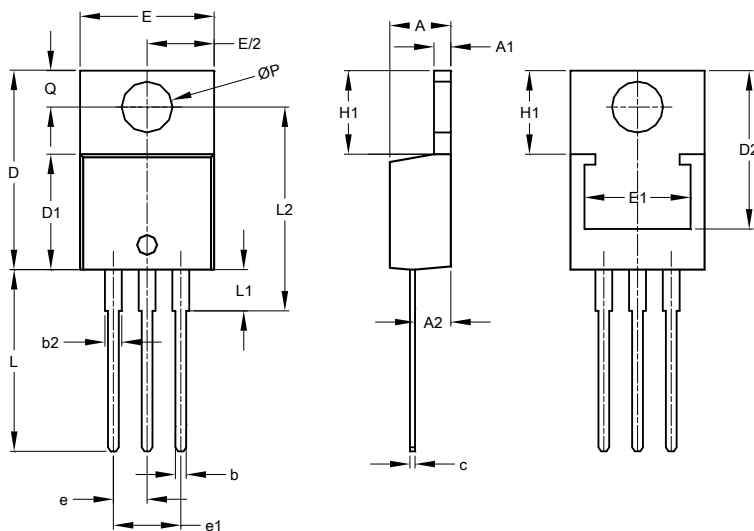
TO220AB
