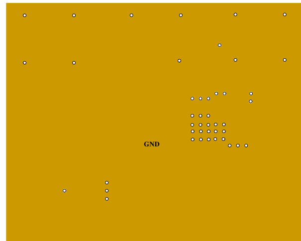
Inner1 Layer
