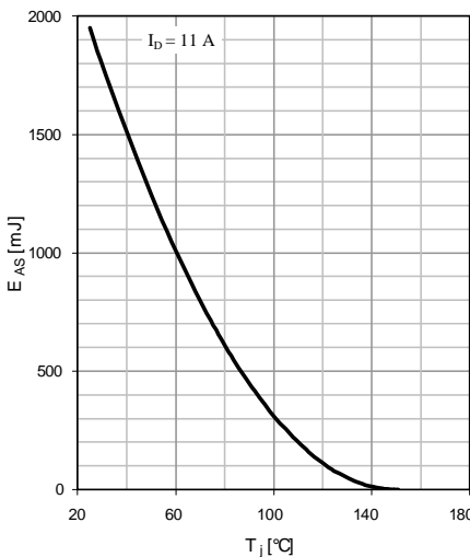
Fig. 9 Avalanche energy
