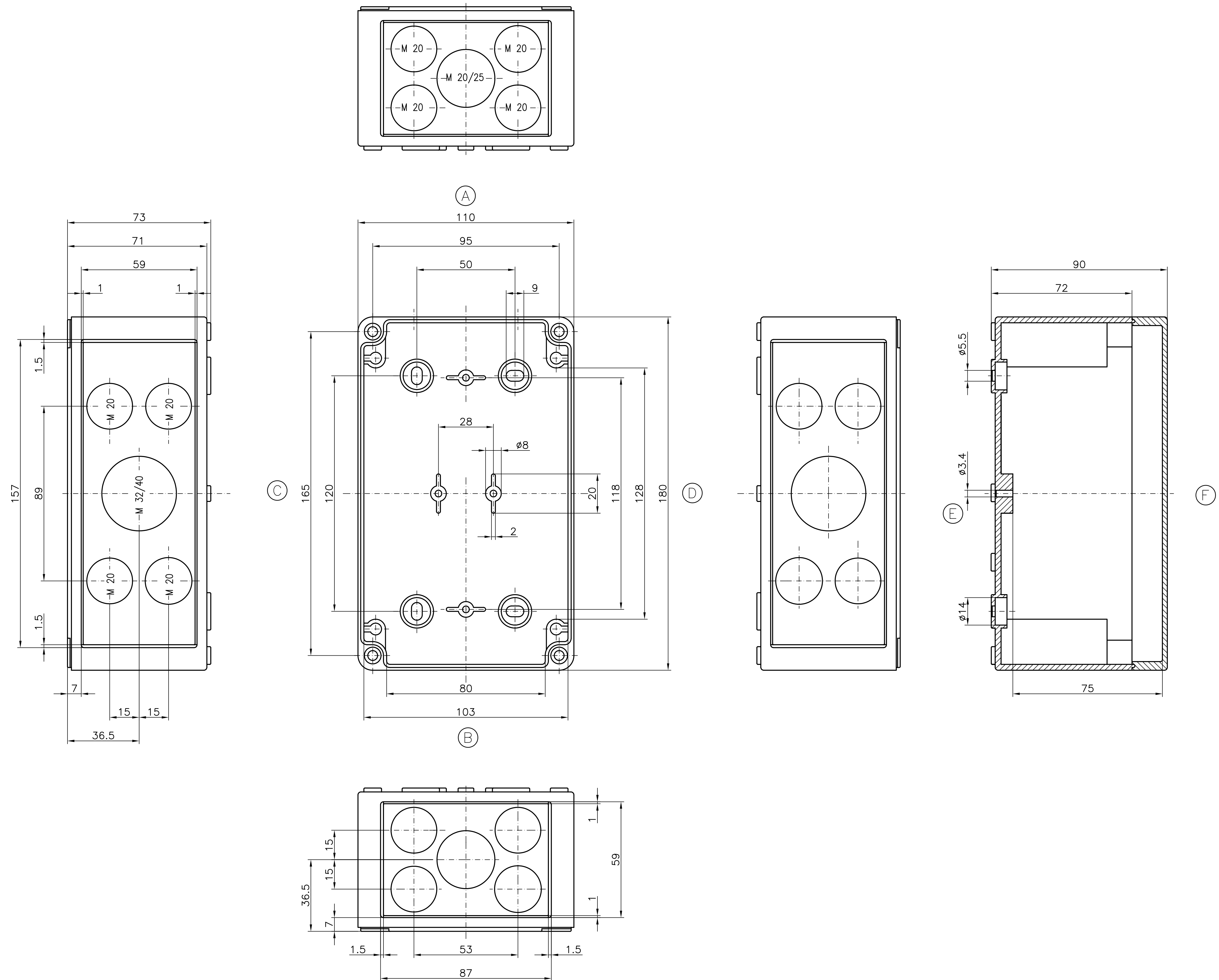
Kompaktgehäuse PCI 08-9M Bestell-Nr. 60.111815
