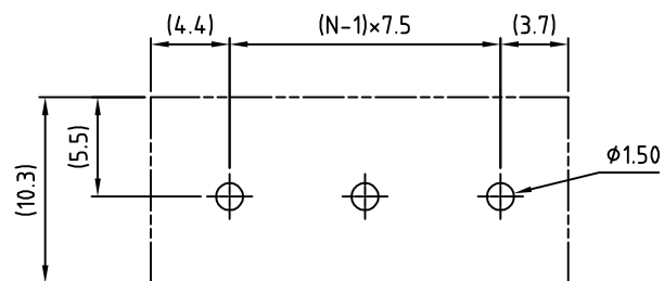
P.C.B LAYOUT
