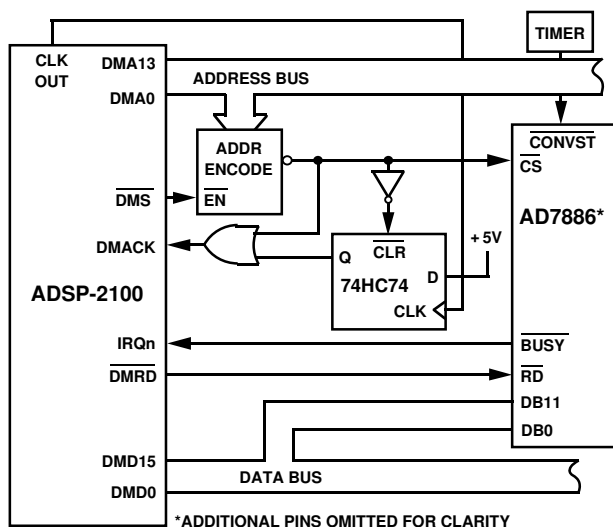
Figure 17. AD7886–ADSP-2100 Interface
