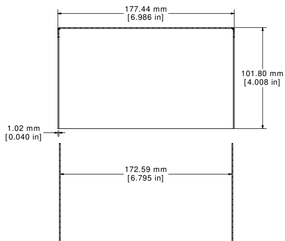
SECTION ZZ-ZZ
