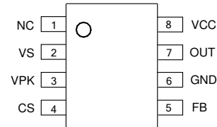
SO-8
