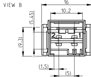
VIEW B TURNED Ansicht B gedreht
